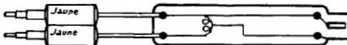
SSY-SONDE SYMETRIQUE 300 OHMS
