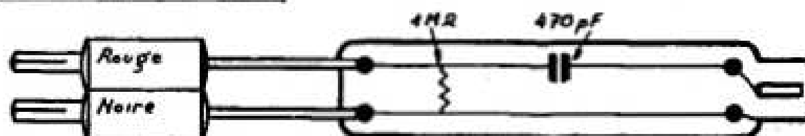
SCO SONDE CONDENSÉE
